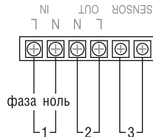
Рис. 15. Пример подключения соединительных проводов к терморегулятору CALEO
